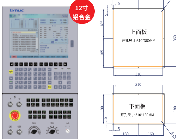
上/下面板外形尺寸分别为: 330*380mm / 330*200mm
