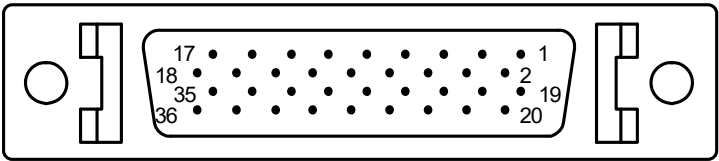
图 3-5 CN1/2/3/4/5/6 接口示意图
