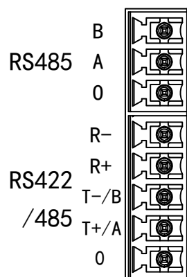
图 3-10 串口输入接口
