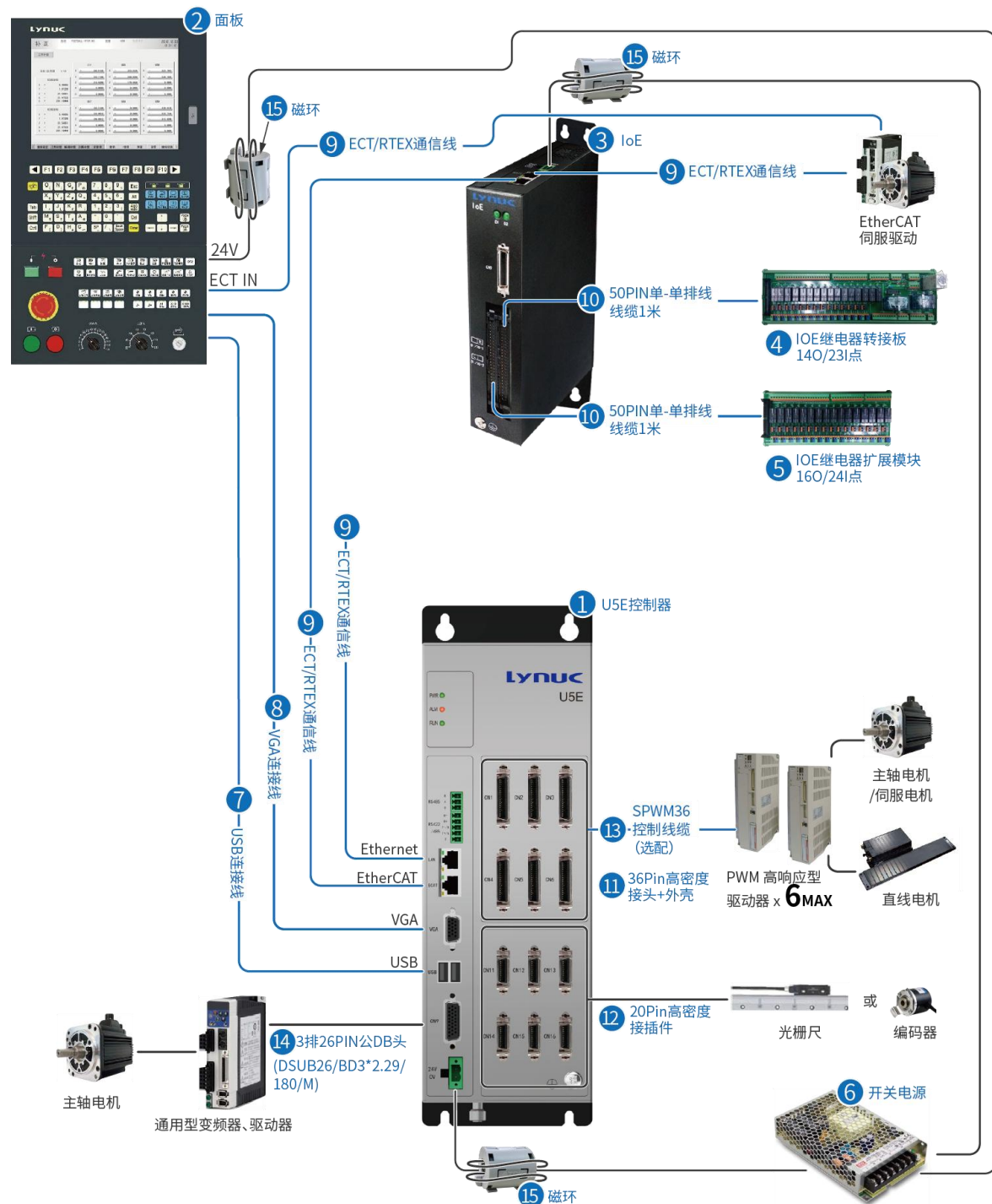
图 3-2 U5E 控制器连接示意图
