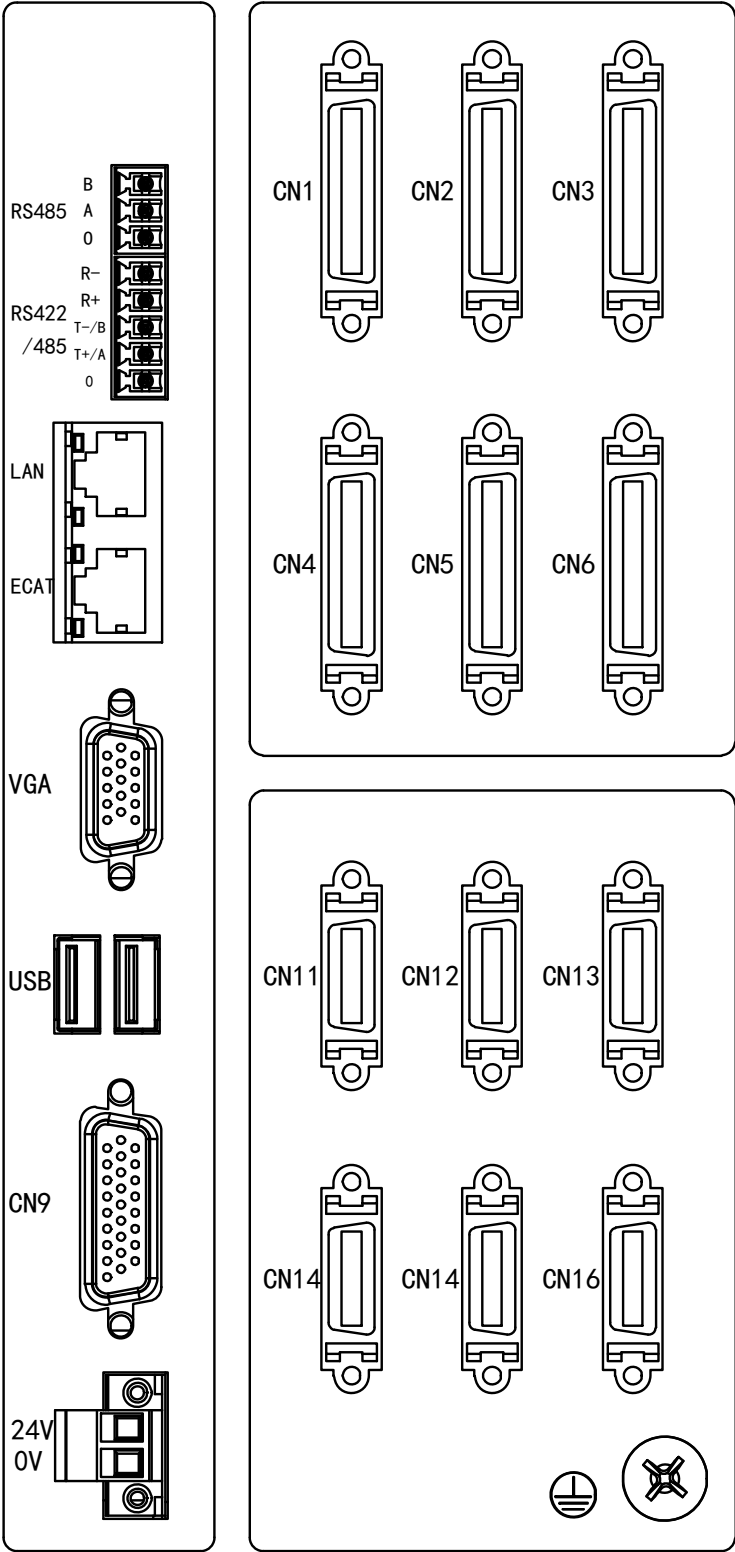
图 3-4 U3E/U5E/U6A 控制器各轴接口图
