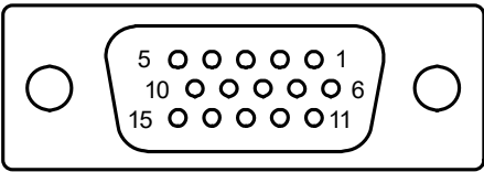
图 3-8 VGA 接口示意图
