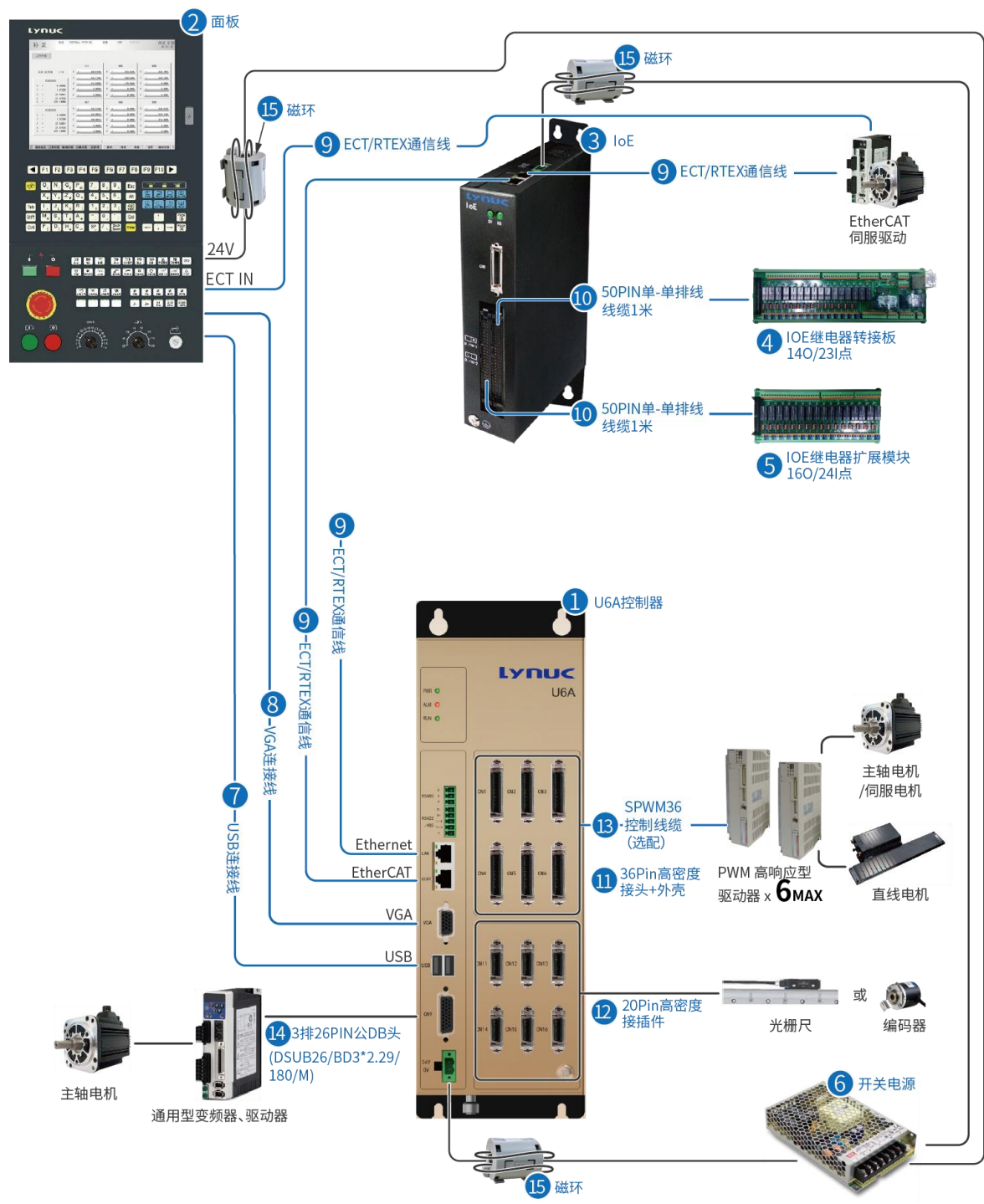
图 3-3 U6A 控制器连接示意图
