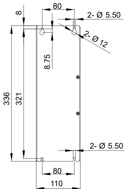
图 4-2 安装尺寸图-1
