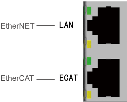
图 3-11 EtherCAT 和 EtherNET 网络接口
