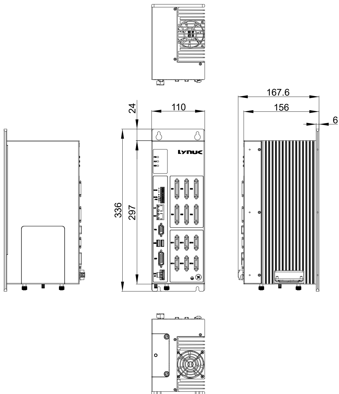
图 4-1 产品外尺寸
