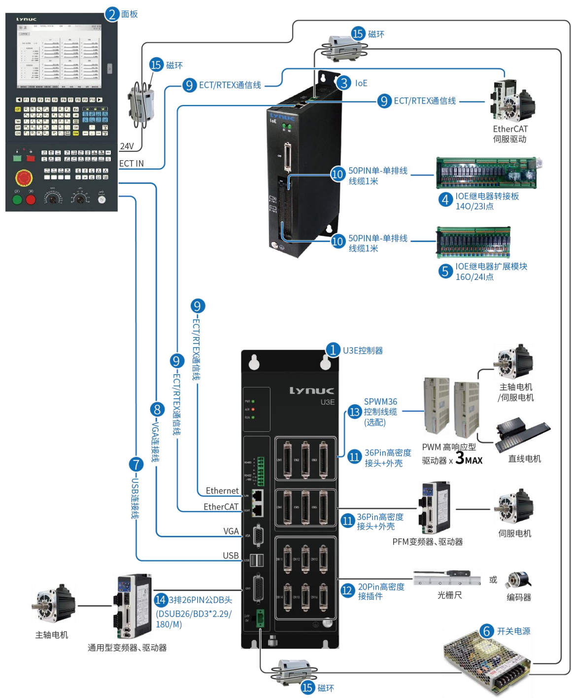
图 3-1 U3E 控制器连接示意图
