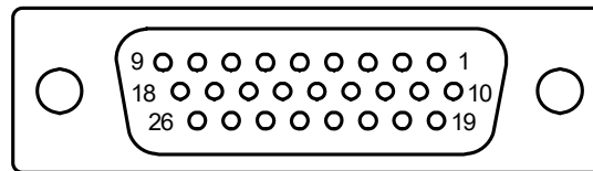
图 3-7 CN9 接口示意图
