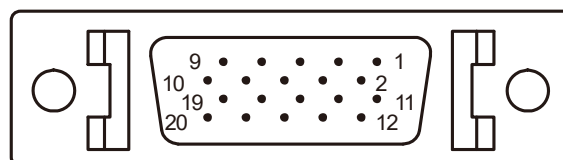
图 3-6 CN11/12/13/14/15/16 接口示意图
