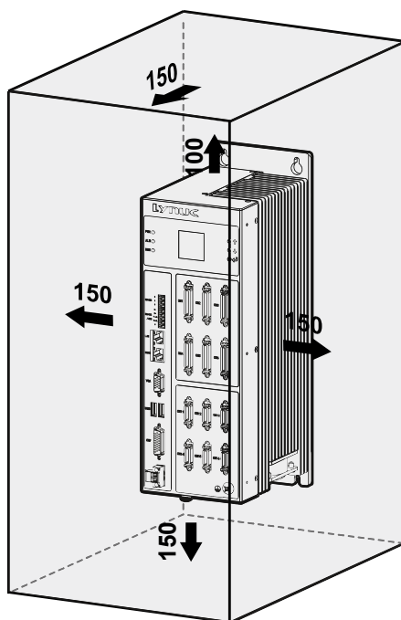
图 4-3 安装尺寸图-2
