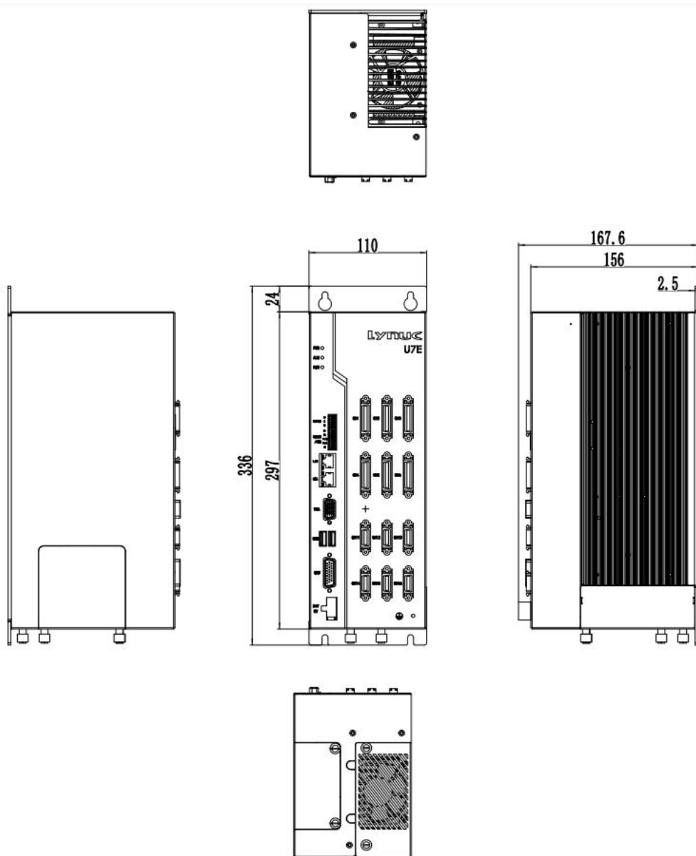
图 4-1 产品外尺寸
