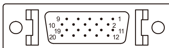
图 3-5 CN11/12/13/14/15/16 接口示意图
