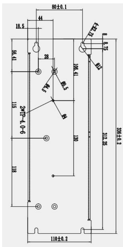
图 4-2 安装尺寸图-1
