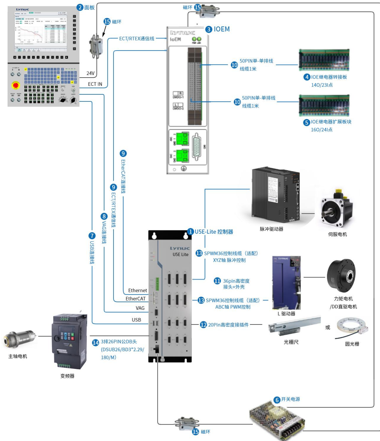
图 3-1 U5EL 控制器连接示意图
