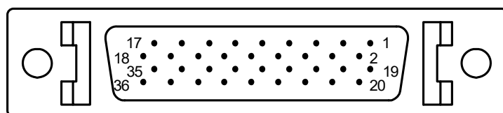
图 3-4 CN1/2/3/4/5/6 接口示意图
