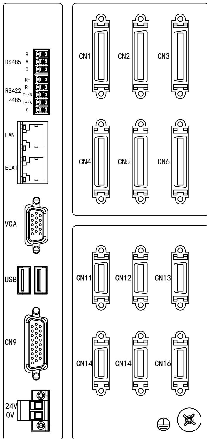
图 3-3 U5LE/U7E 控制器各轴接口图
